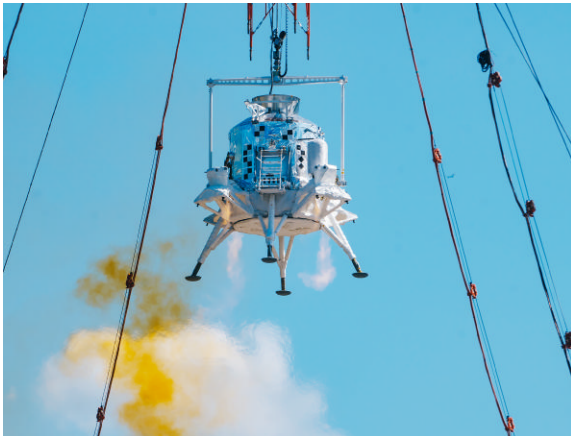
揽月月面着陆器在地外天体着陆试验场进行测试(资料照片) 新华社 发(张斌 摄)
