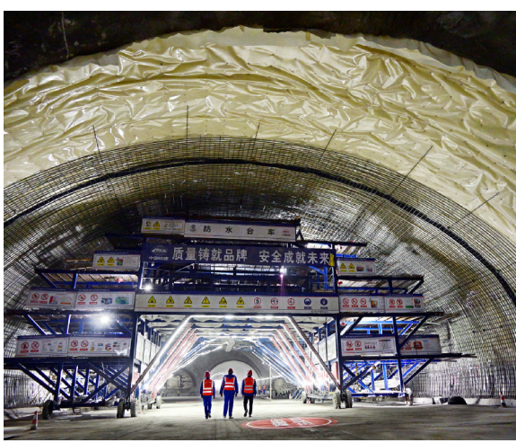
唐山路隧道右线在进行二次衬砌施工作业（3月28日摄）。3月28日，青银高速公路增设唐山路互通及连接线工程唐山路隧道贯通，为全线通车打下坚实基础。据介绍，该隧道全长1551米，双向双洞8车道，最大开挖跨度31.8米，最大开挖断面447.62平方米，是我国最大开挖断面市政交通隧道。
