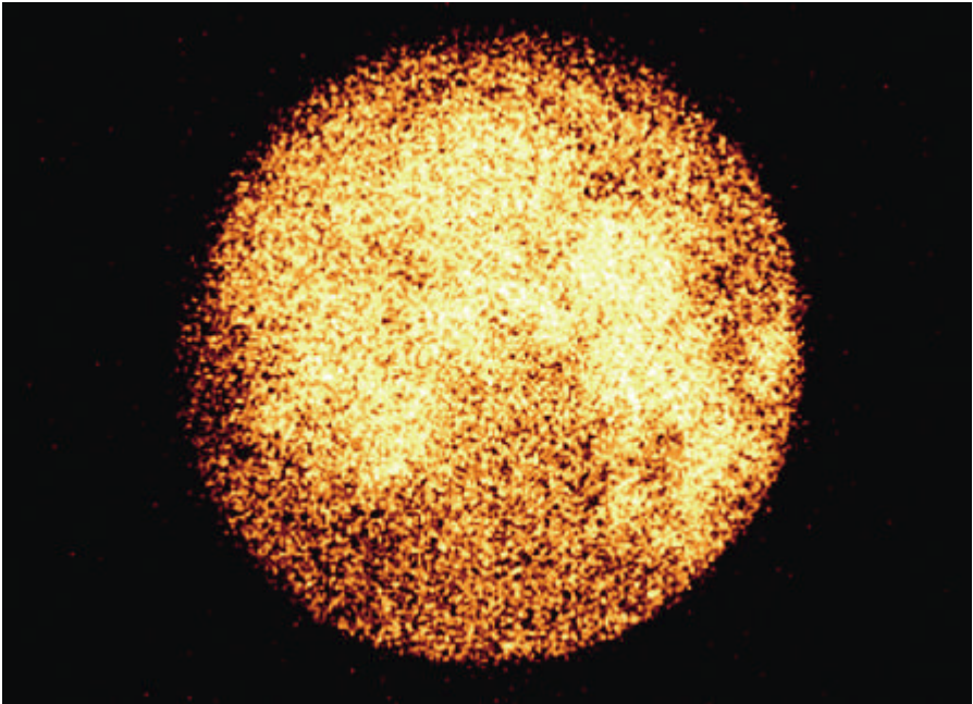
爱因斯坦探针卫星“风行天”X射线望远镜所拍摄的月球X射线图像
