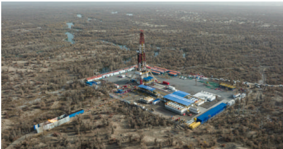
11月15日拍摄的中国石化“深地一号”跃进3-3XC井(无人机照片)
